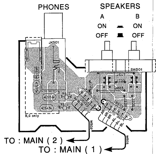
P.C.B. MAIN ( 3 )
